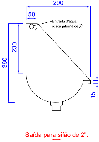
Vista lateral
