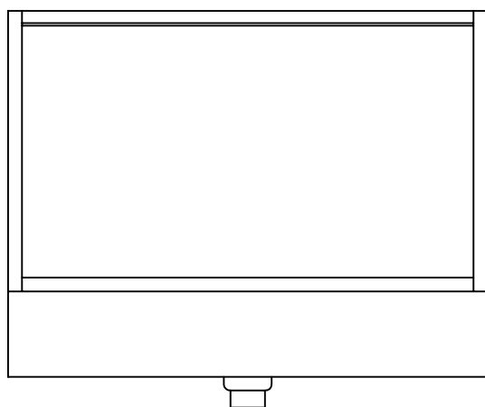
Vista elevação
